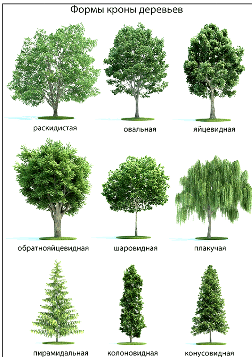
Рис. 3. Форма кроны деревьев ( http://www.google.ru/imgres?imgurl )
