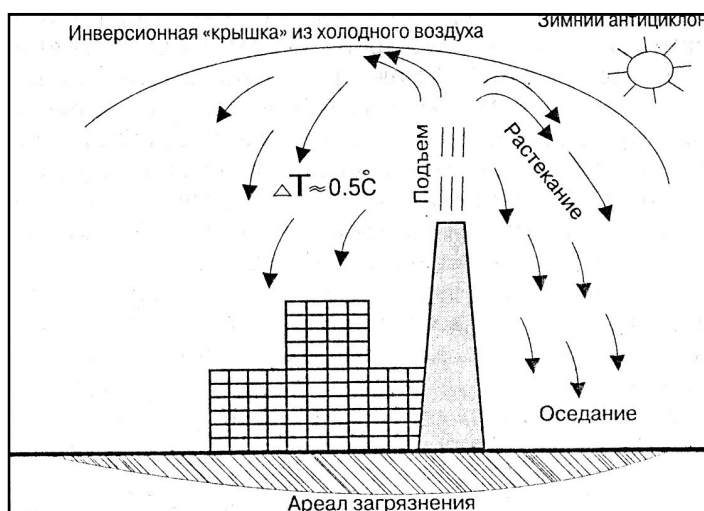
Рис. 1. Формирование ареала загрязнения в условиях зимнего антициклона (Колбовский, 2006)
