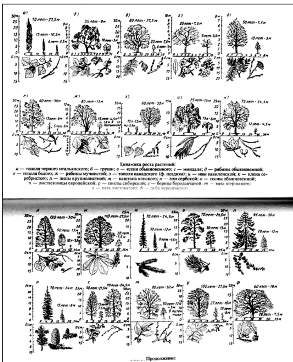
Рис. 2. Жизненные параметры разных видов деревьев
